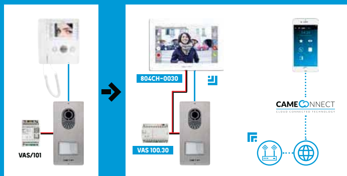
Alimentazione unica XTS e posto esterno
