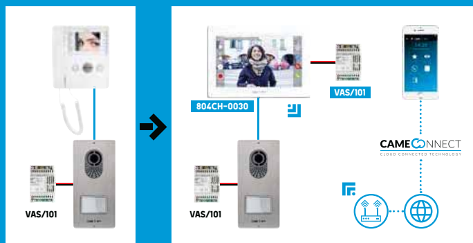
Alimentazione separata XTS e posto esterno
